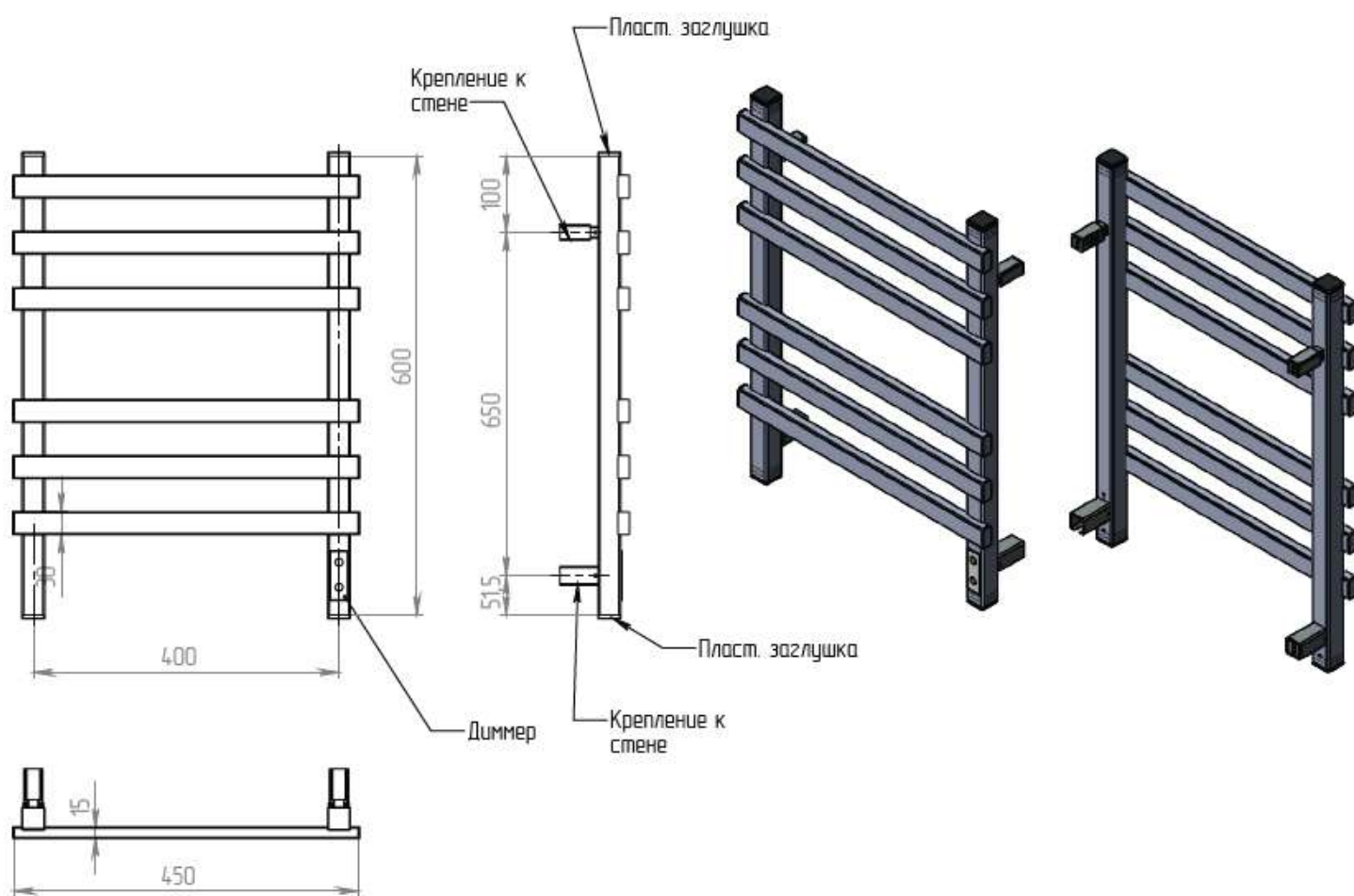
Электрический полотенцесушитель Двин Серии PLAZA NEO N PLAZA NEO 600x400
